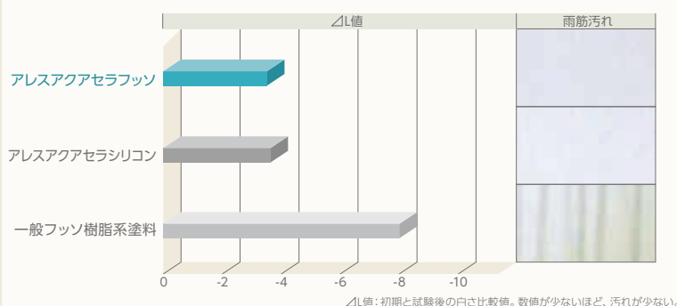
白塗料における屋外バクロ6ヵ月の \Delta L 値と塗膜状態
